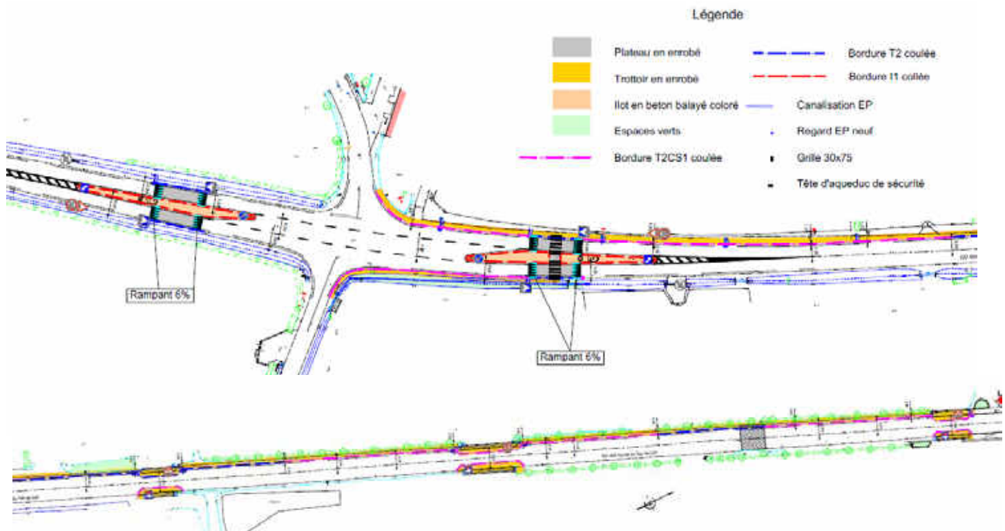
Etude de voirie - le Bourg - La Croix Caseau
